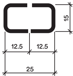
1 Lochreihe
